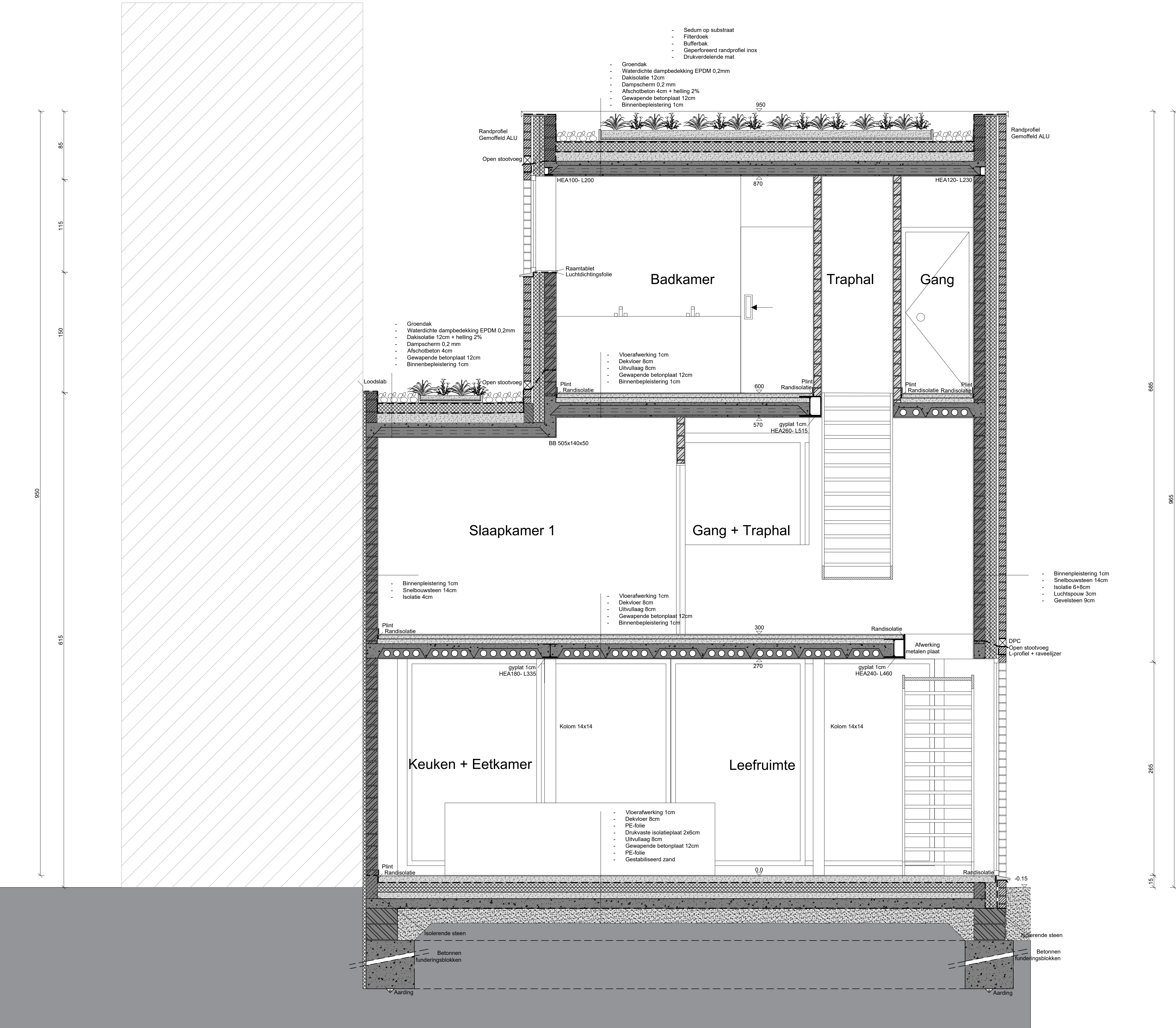
Snedes DD' Schaal 1/25
