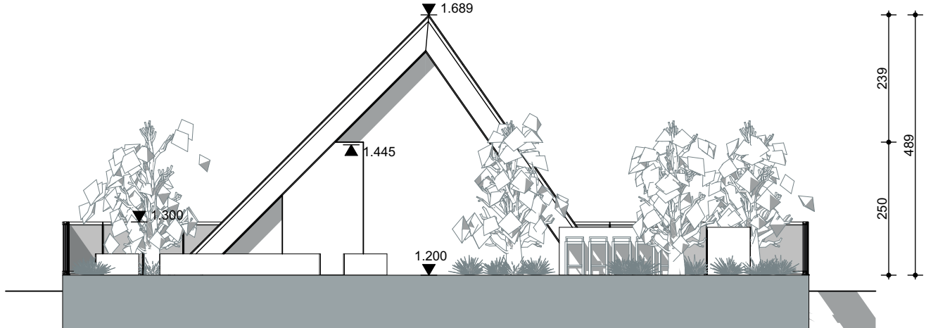
GEVEL D- 1/100
