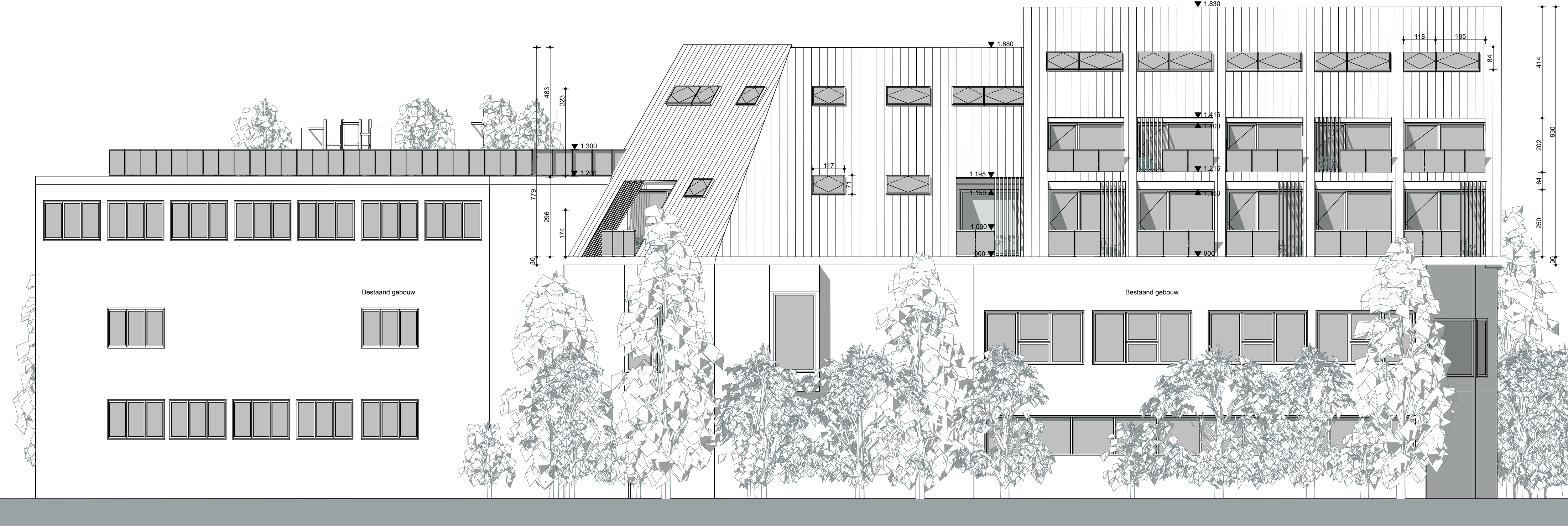
GEVEL A- 1/100
