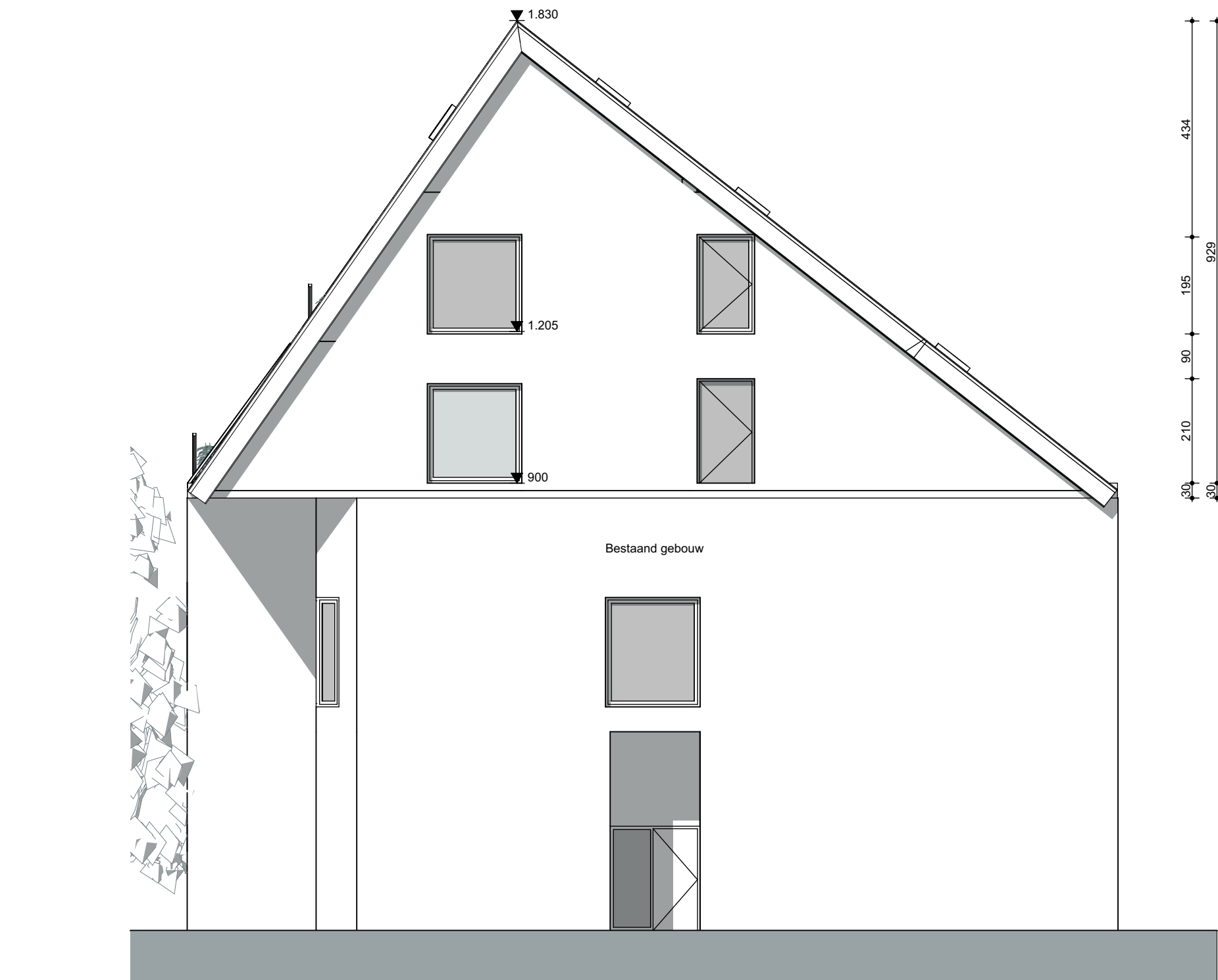
GEVEL B- 1/100
